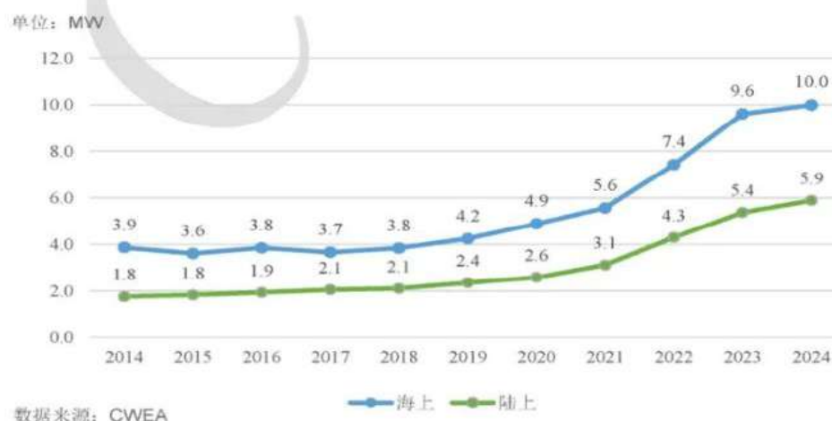
图 2 2014-2024 年中国风电新增陆上和海上风电机组平均单机容量
