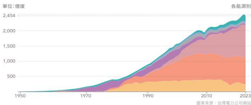
2023 年發購電量結構
